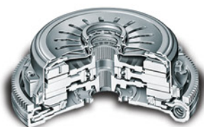
Dupla Embreagem
